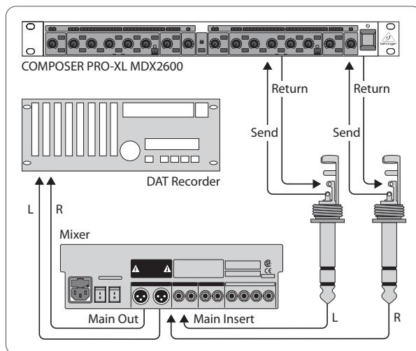
图 4.2: 用 MDX2600 压缩总混音信号
