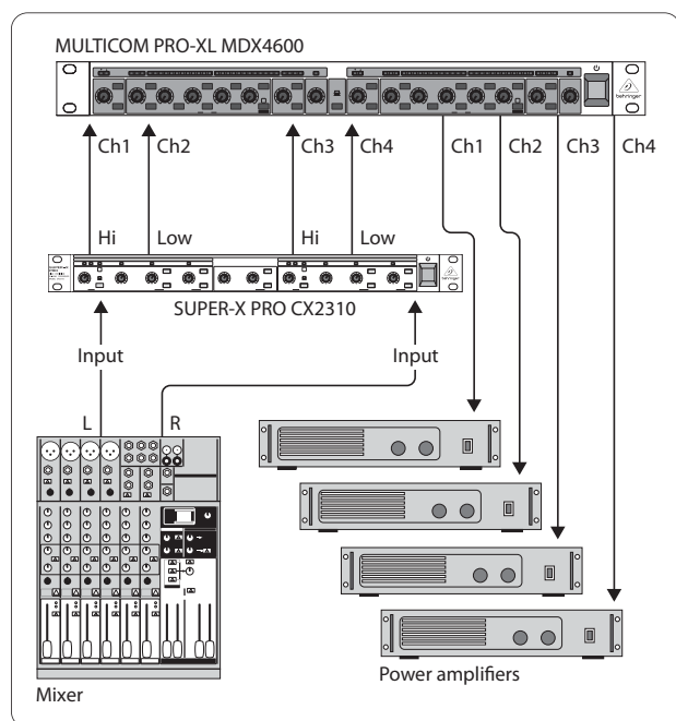
图 4.3: MDX 4600 多频段压缩
