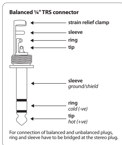
图 5.3: 1/4" TRS 接口
