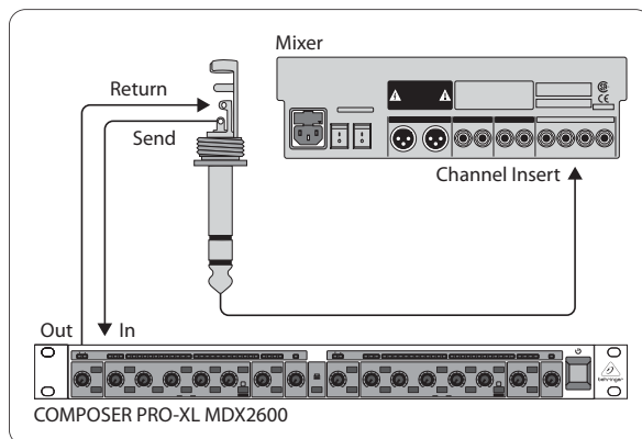
图 4.1: 将动态处理器插入至输入路径
