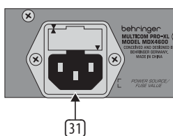
图 2.7: 电源及保险丝
