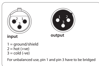
图 5.1: XLR 接口
