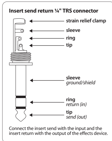
图 5.4: 1/4" TRS 接口
