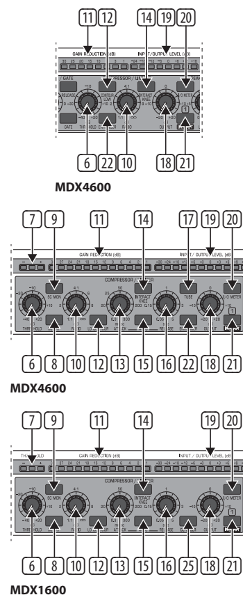
图 2.3: 压缩器区控制键
